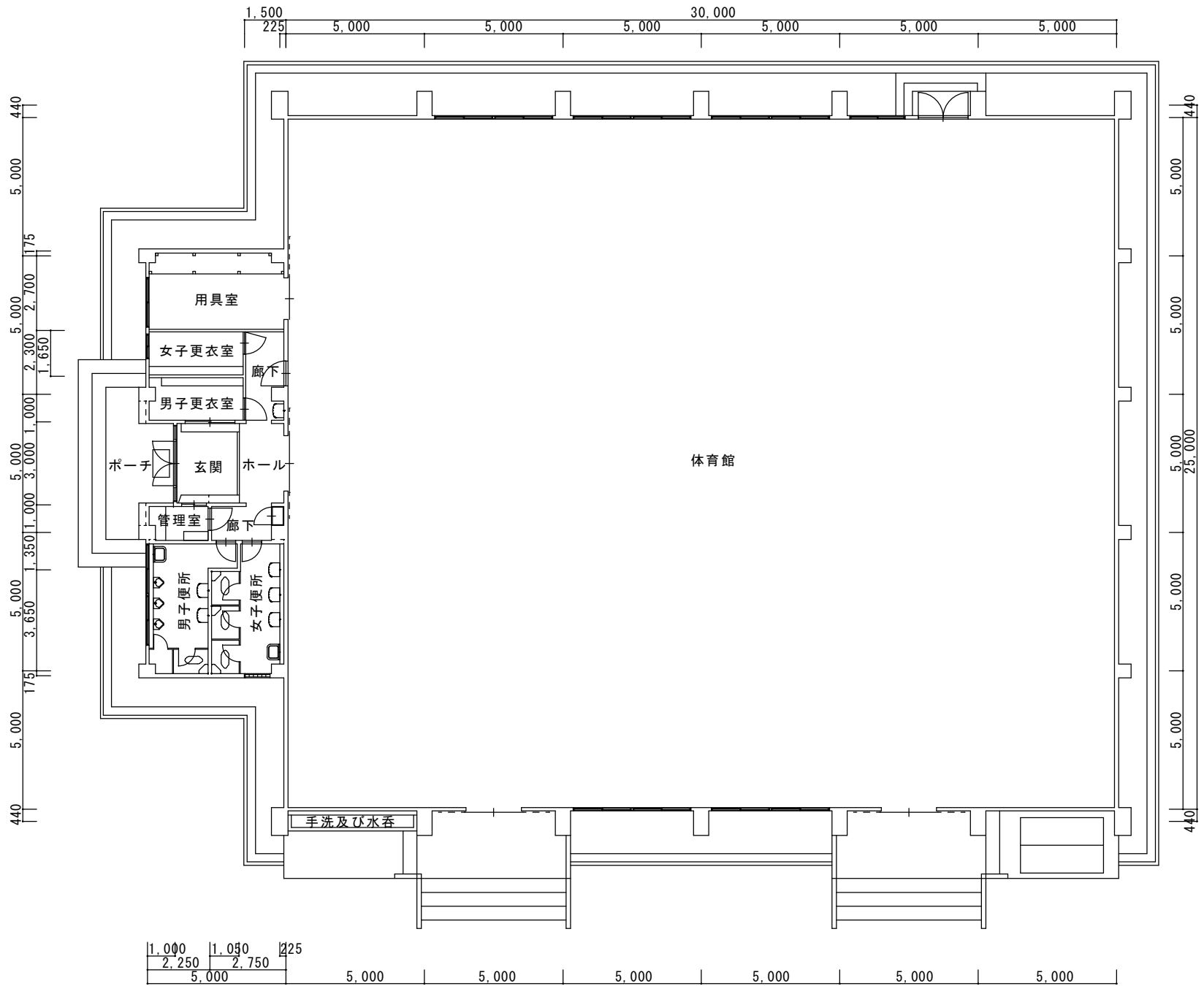
1階平面図 1 : 100
