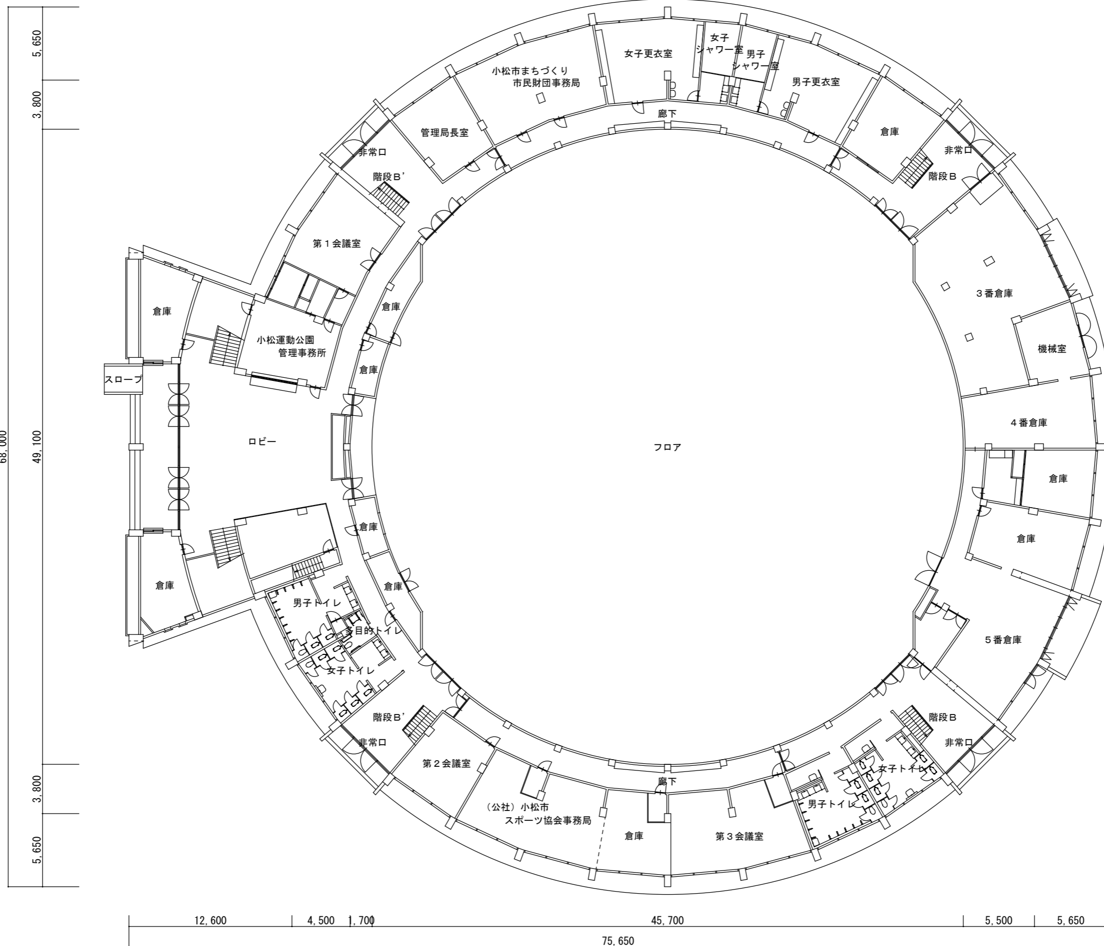
1階平面図 1/300
